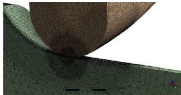
Канечна-элементная мадэль кантактнага ўзаемадзеяння
