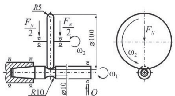
Прынцыповая схема сістэмы «ролік – вал»
